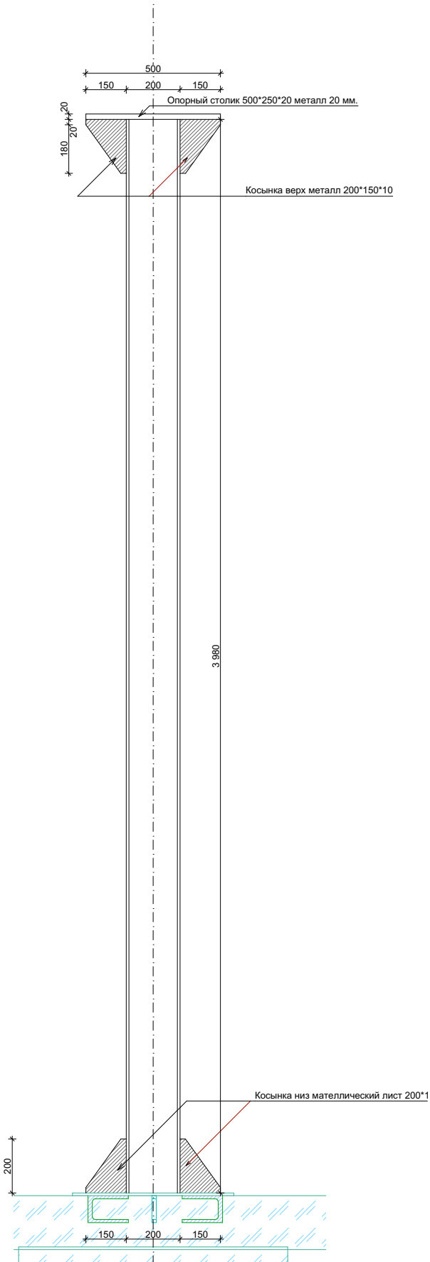
Разрез 7-7
